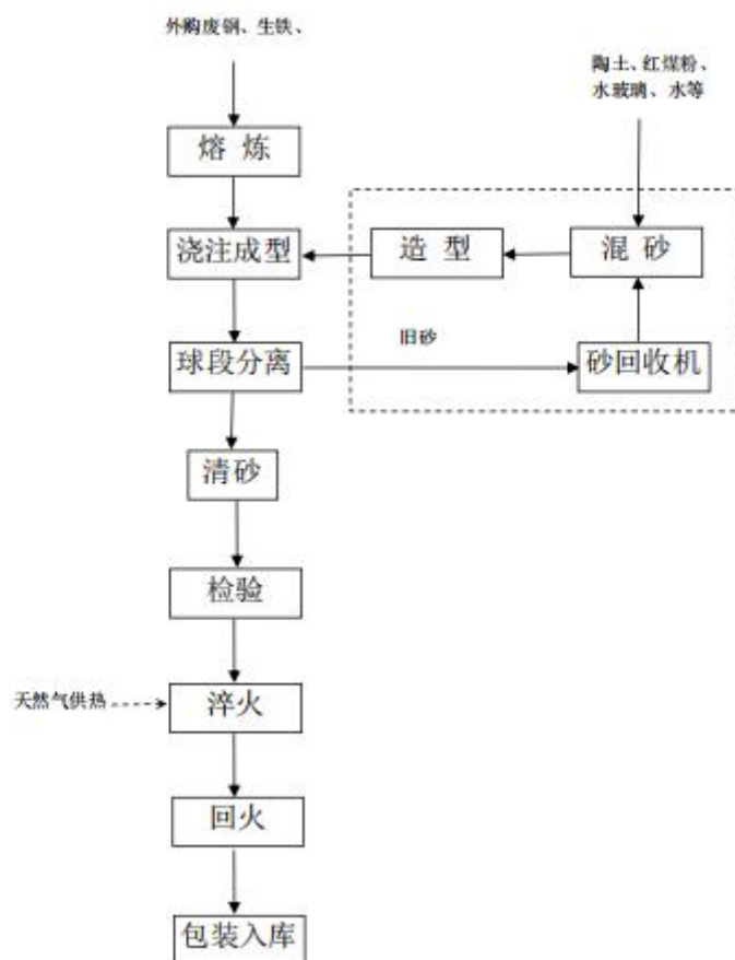
图 3-1 生产工艺流程图
