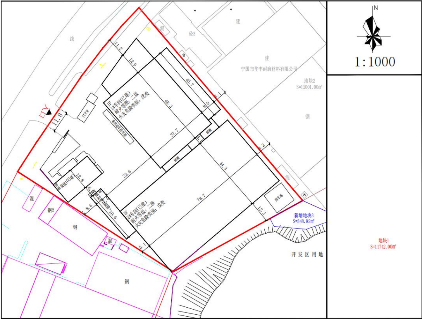
图 3-3 企业厂区平面布置图
